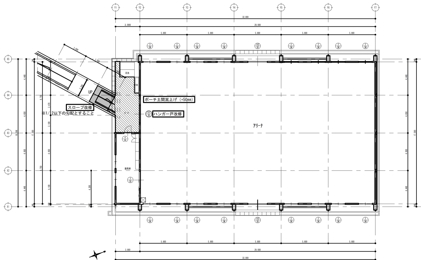
【体育館】改修後1階平面図 S=1:100
