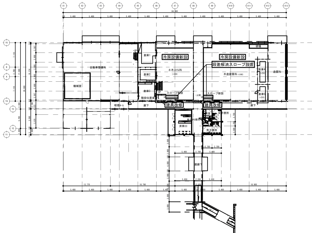
【実習棟】改修後1階平面図 S=1:200
