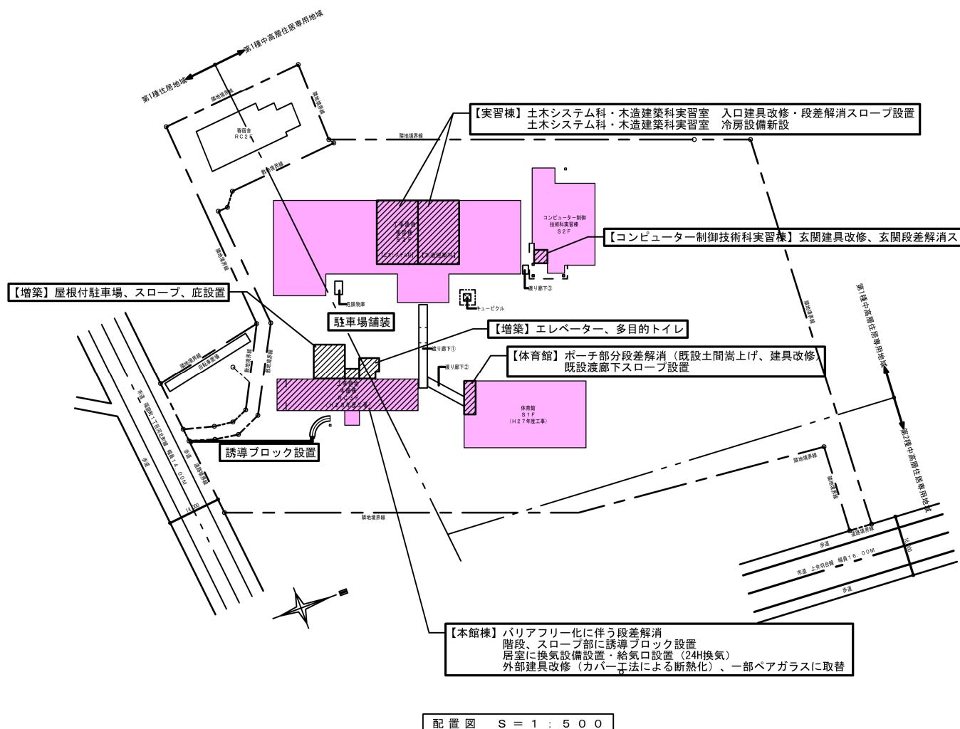
配置図 S = 1 : 5 0 0
