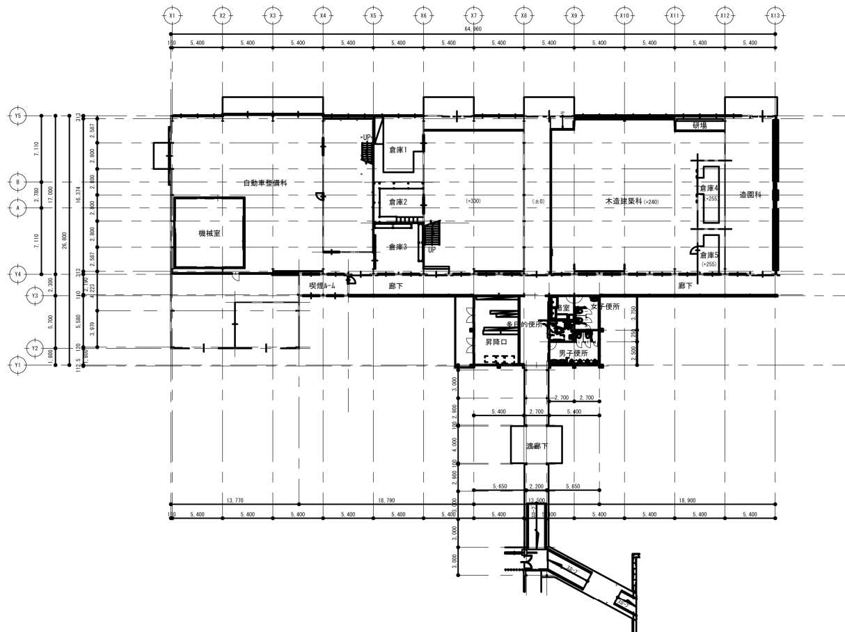
【実習棟】改修前1階平面図 S=1:200
