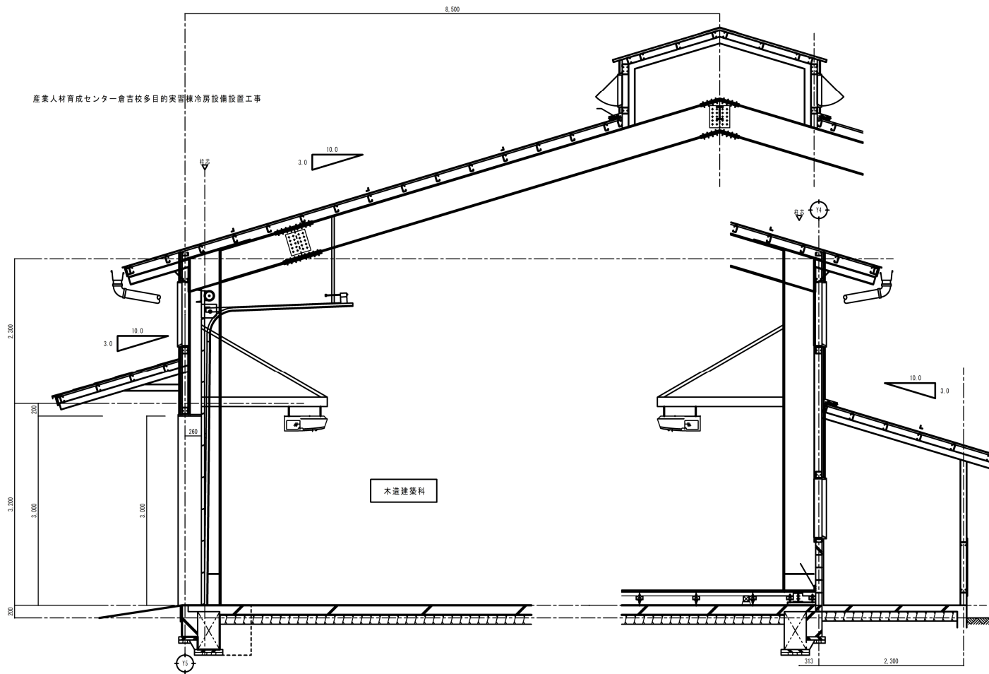
木造建築科 エアコン設置参考図
