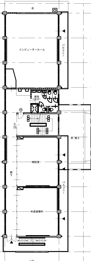
【本館棟】改修前2階平面図 S=1:100
