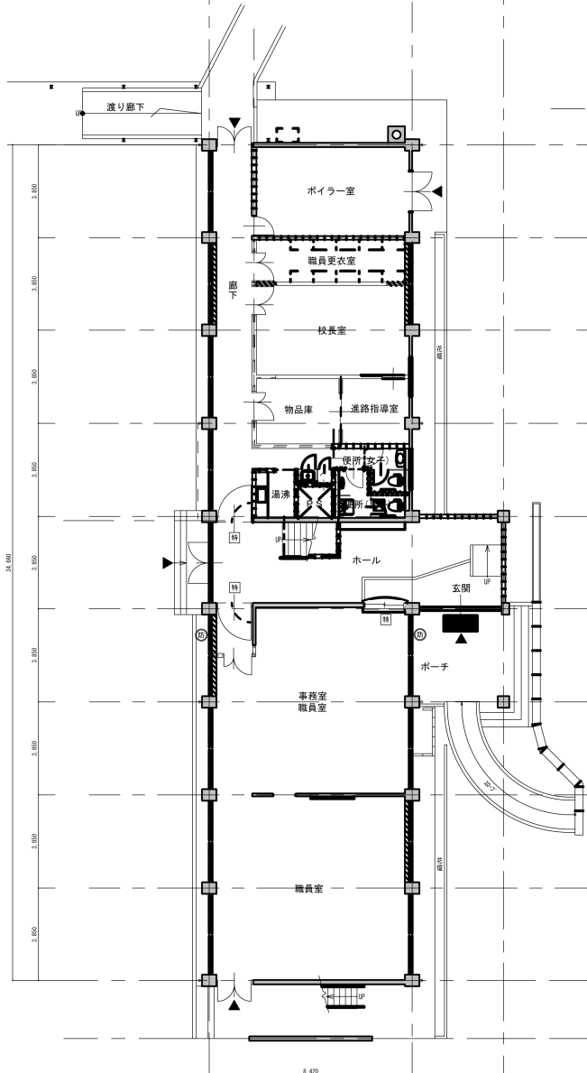
【本館棟】改修前1階平面図 S=1:100
