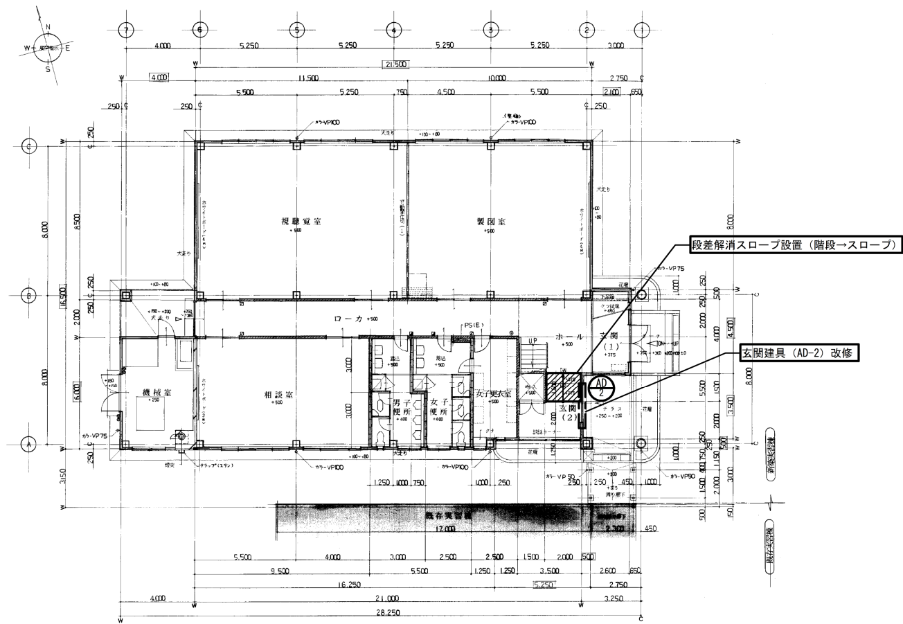
【コンピュータ制御技術科実習棟】改修後1階平面図 S=1:200
