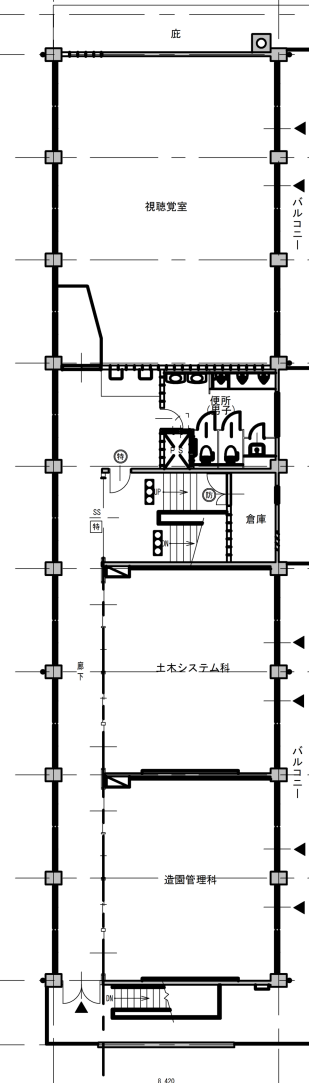
【本館棟】改修前3階平面図 S=1:100
