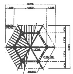
小屋伏図 S = 1/100
