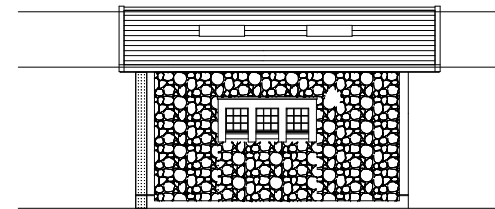
【南立面図 S=1/150】
