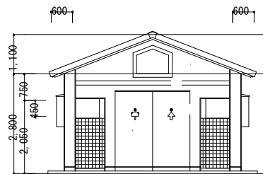
【東立面図 S=1/150】
