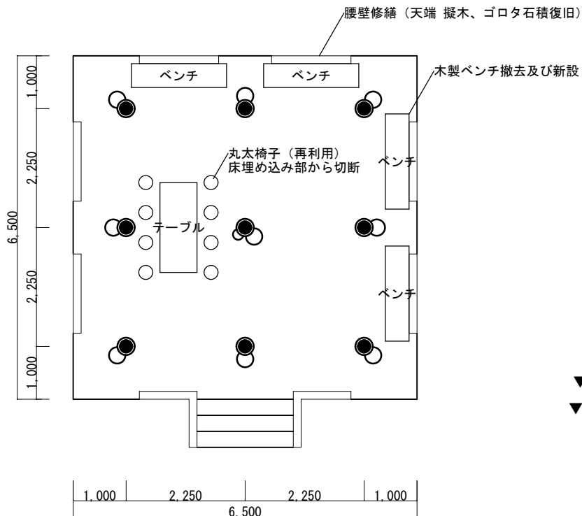
【平面図 S=1/100】
