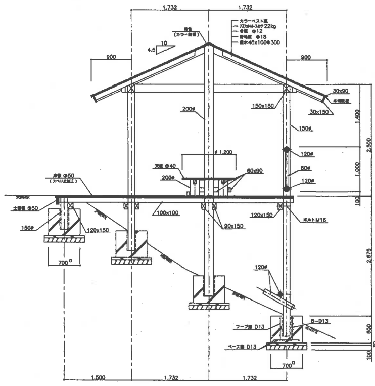
縦断面図 S = 1/30
