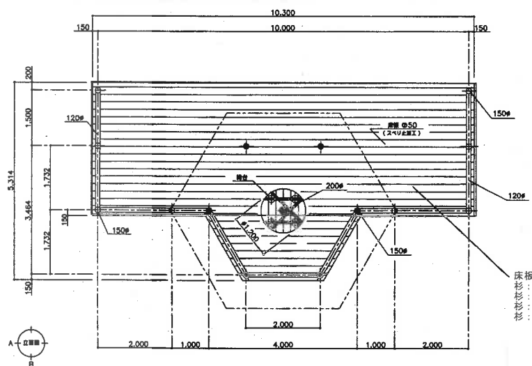
平面図 S = 1/50
