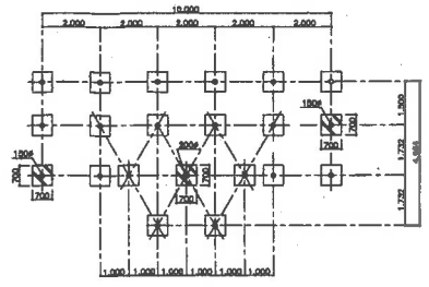
基礎伏図 S = 1/100
