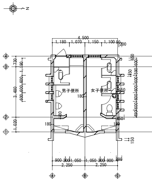
【平面図 S=1/150】
