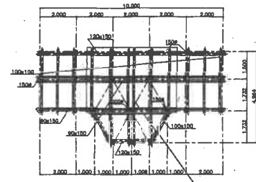
床伏図 S = 1/100
