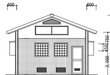
【西立面図 S=1/150】
