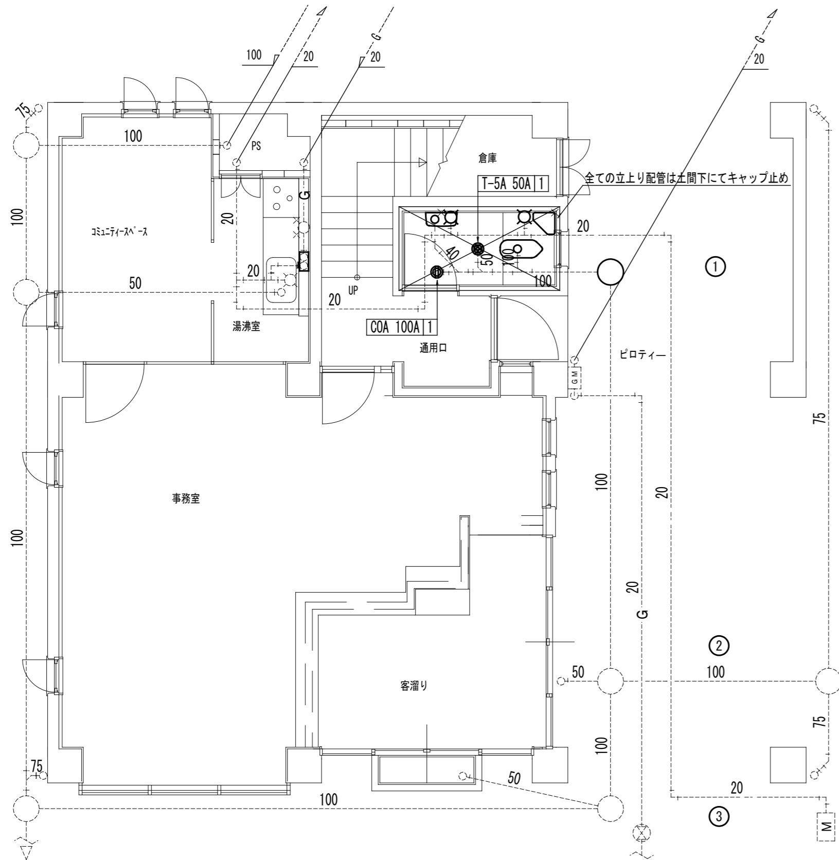
衛生設備 1階撤去図 (改修前) S=1:60
