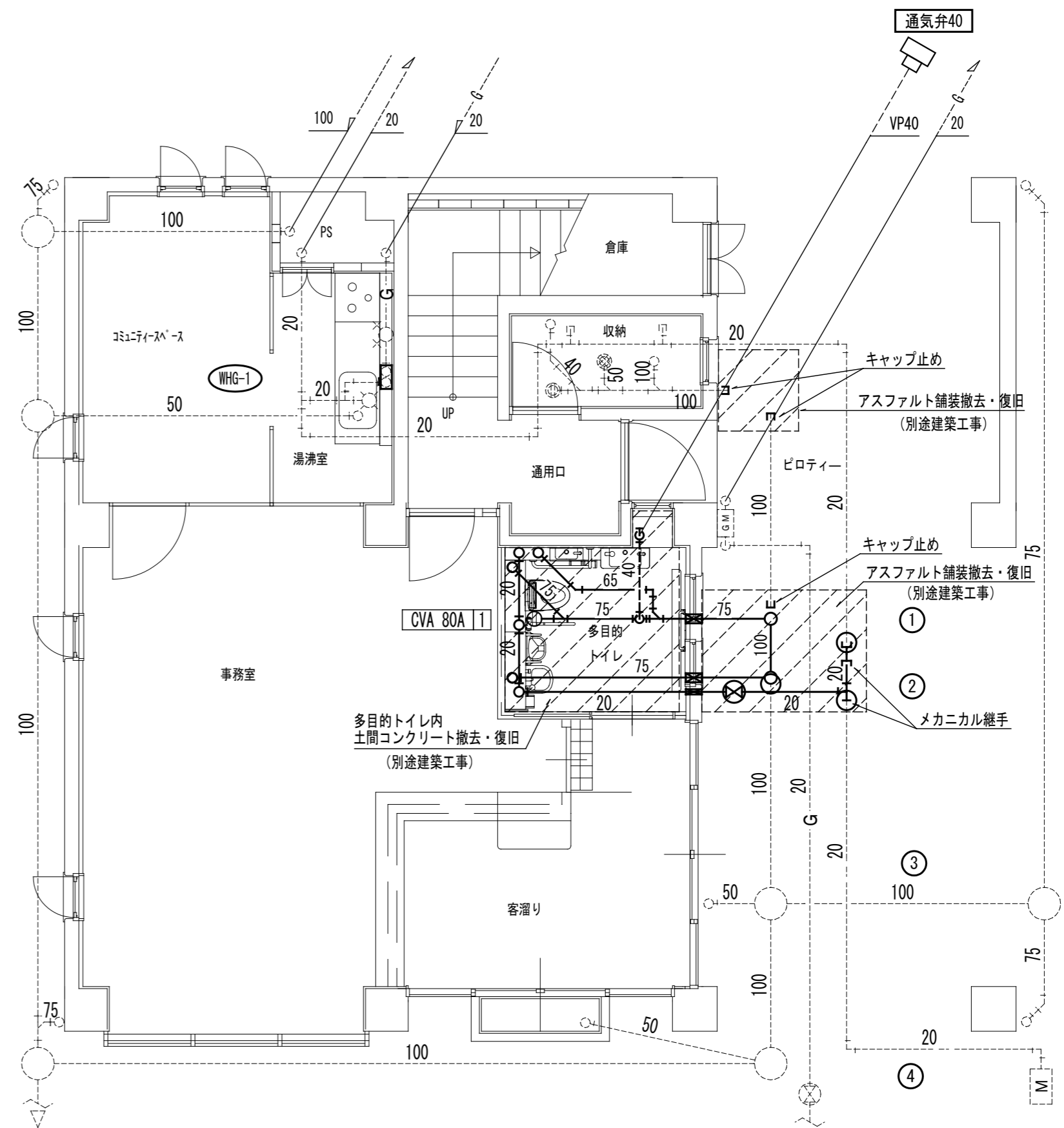
衛生設備 1階改修図 (改修後) S=1:60
