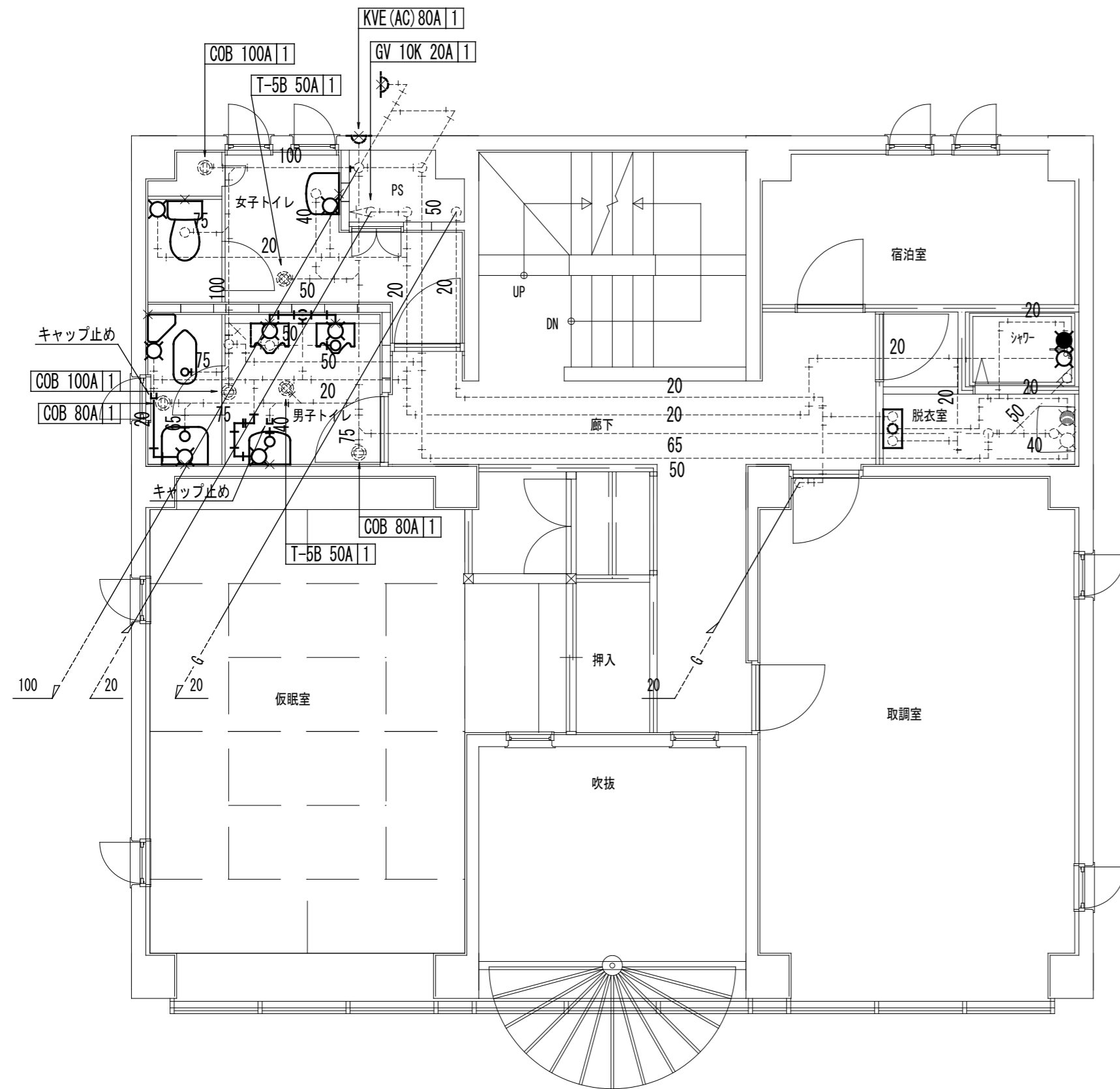
衛生設備 2階撤去図 (改修前) S=1:60
