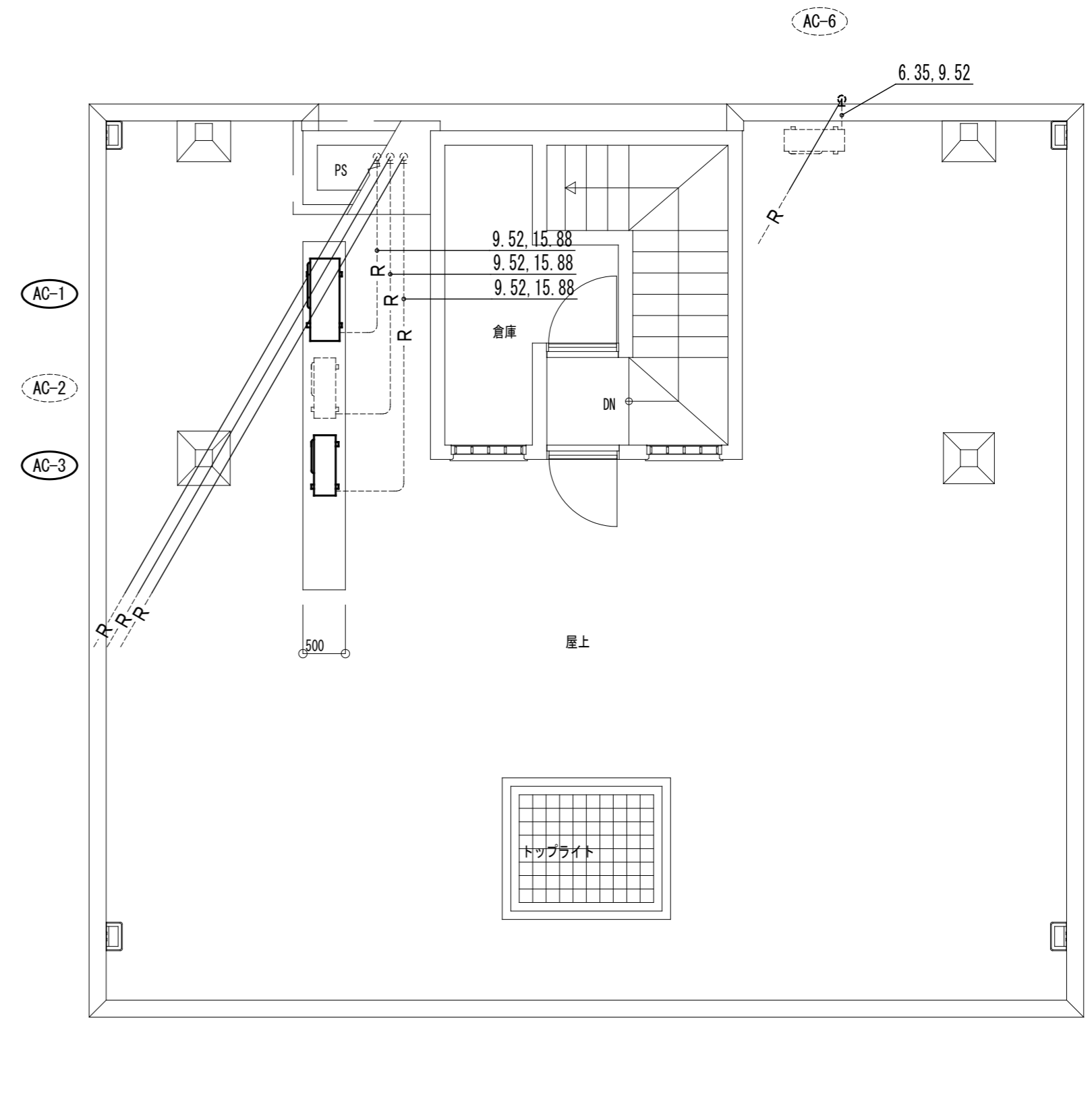
冷暖房・換気設備 3階改修図 (改修後) S=1:60
