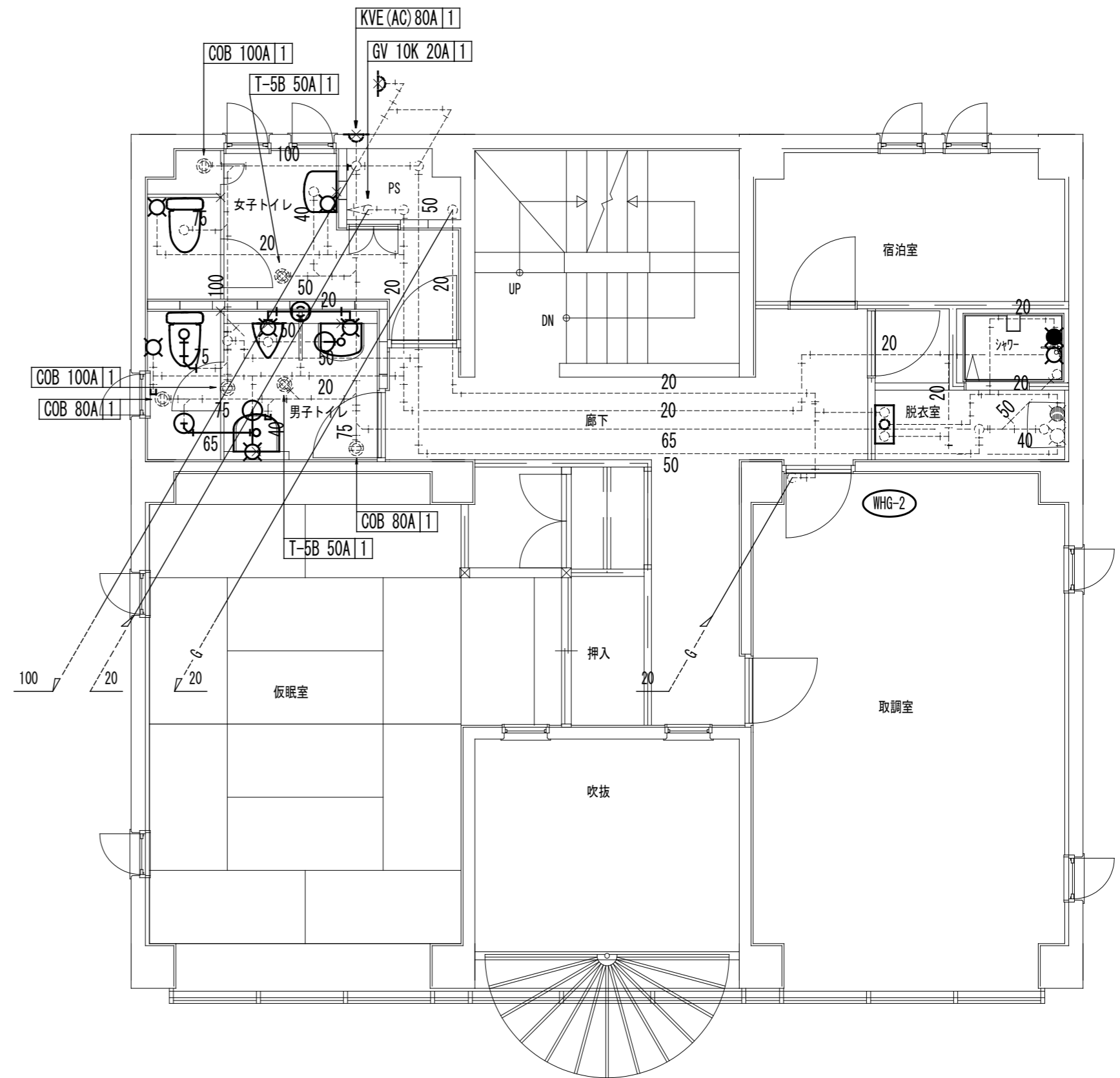
衛生設備 2階改修図 (改修後) S=1:60
