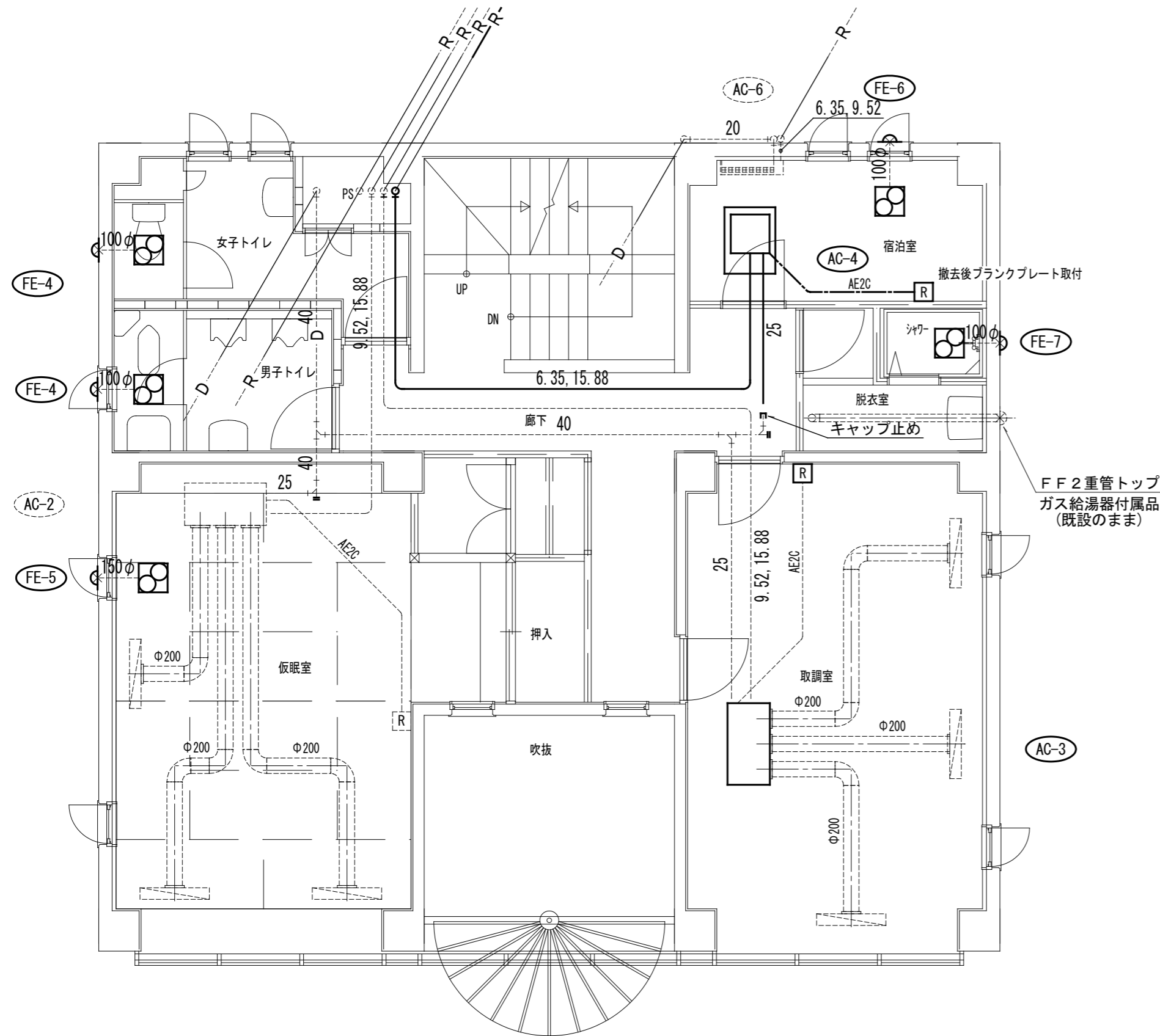
冷暖房・換気設備 2階撤去図 (改修前) S=1:60
