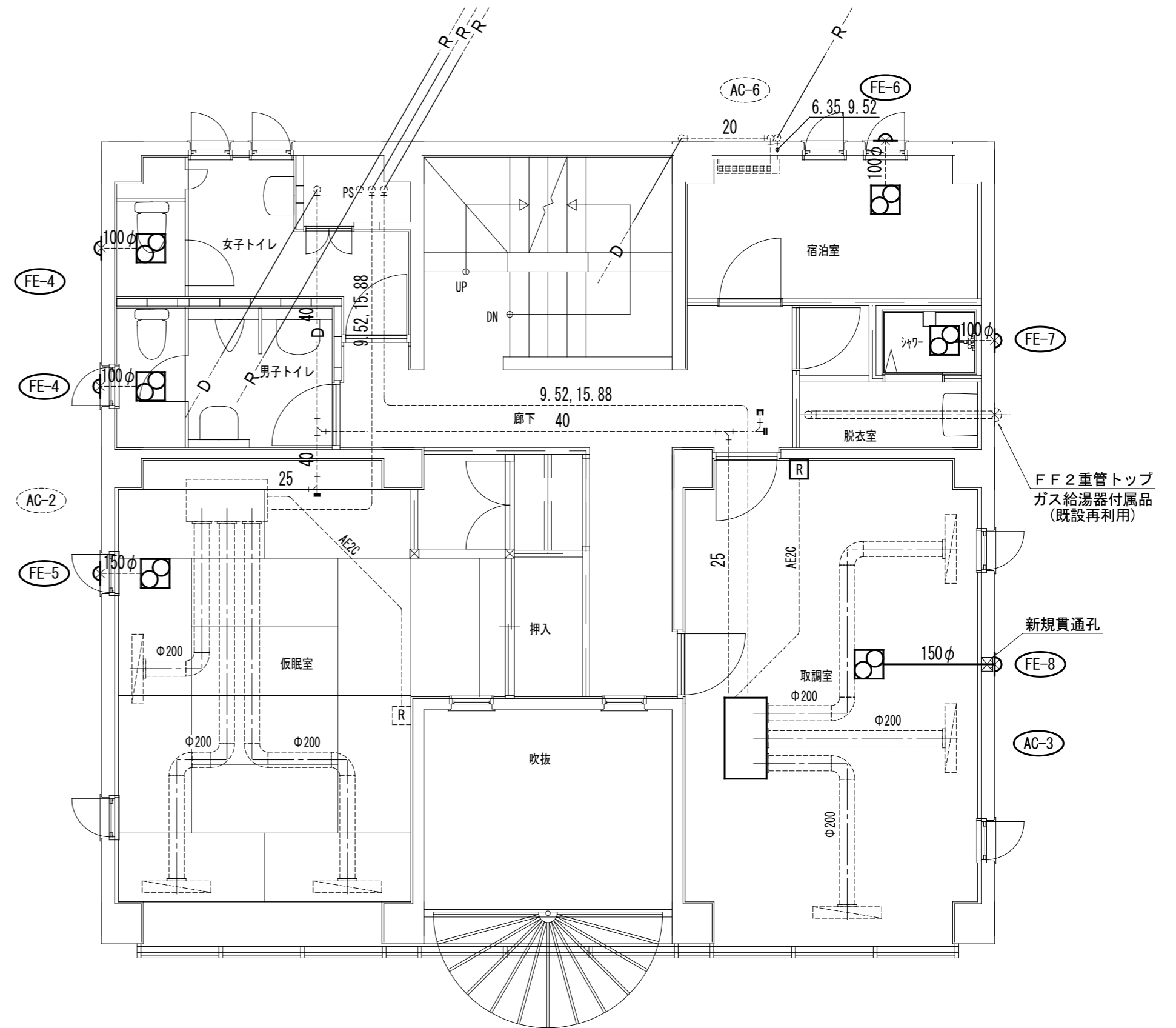
冷暖房・換気設備 2階改修図 (改修後) S=1:60
