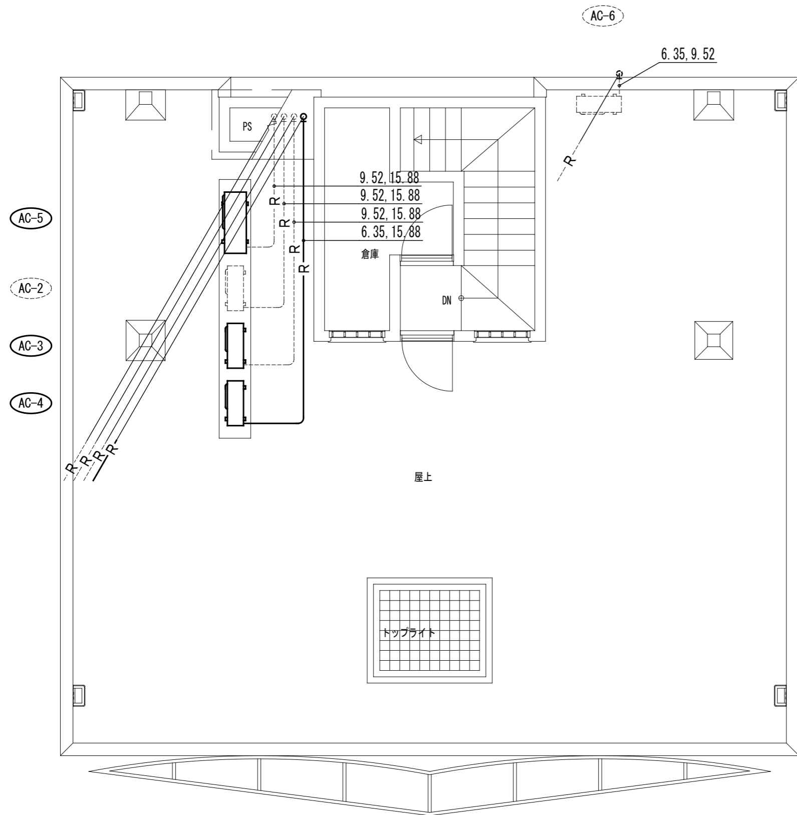
冷暖房・換気設備 3階撤去図 (改修前) S=1:60
