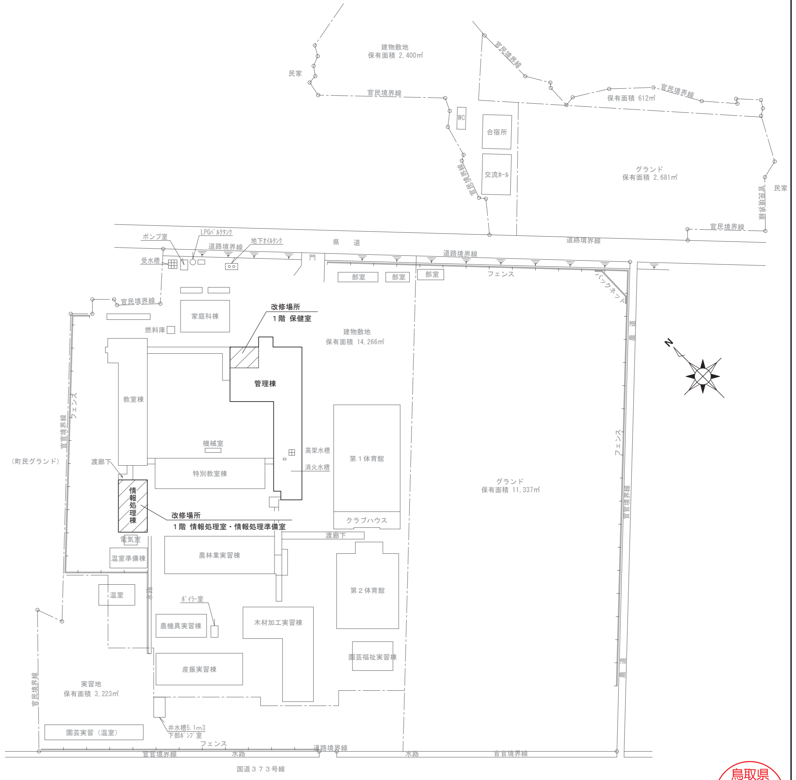
配置図 S=1/800
