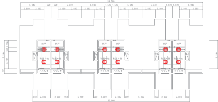
3階平面図 S=1:250
