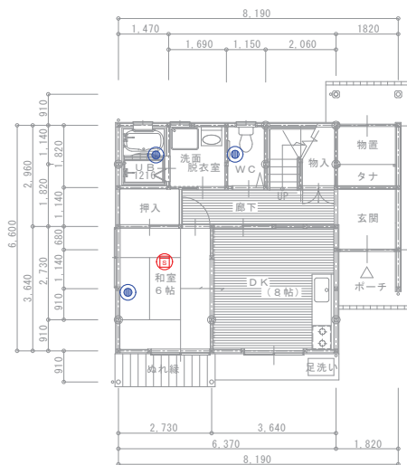
1階平面図 S=1:100
