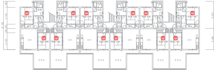
2階平面図 S=1:250
