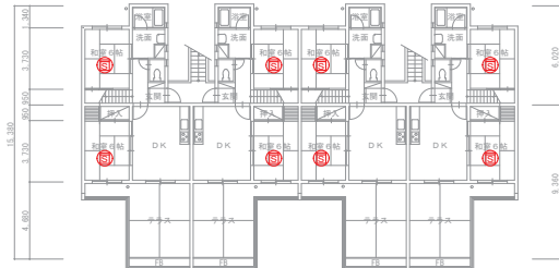
2階平面図 S=1:250
