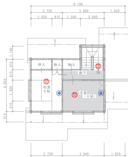
2階平面図 S=1:100
