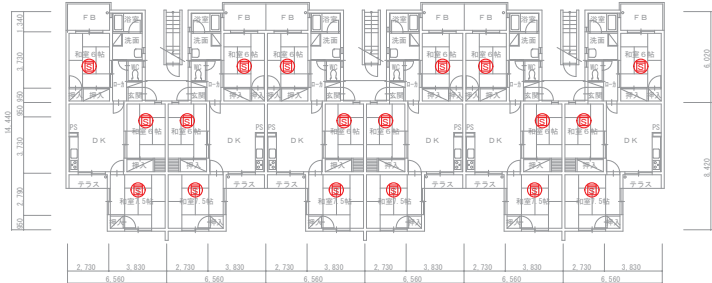
1階平面図 S=1:250
