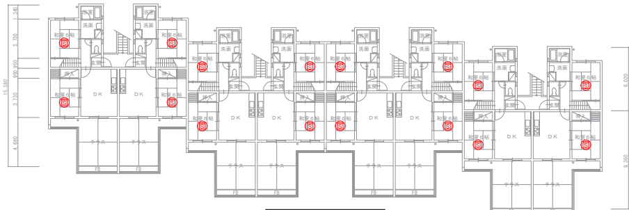
2階平面図 S=1:250
