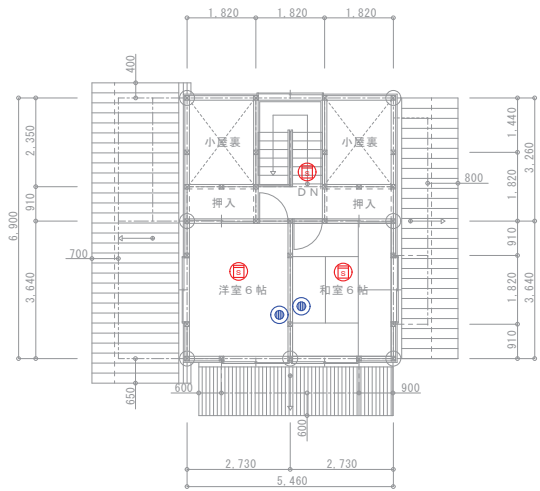
2階平面図 S=1:100
