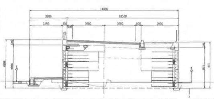
【標準断面図：計画】②（岩倉側）
