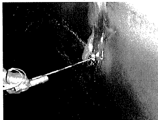
継ぎ目地部より浸入水 (M3-M2 管No.18)
