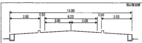
【標準断面図：計画】
