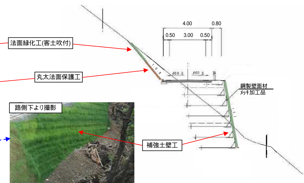
断面図
