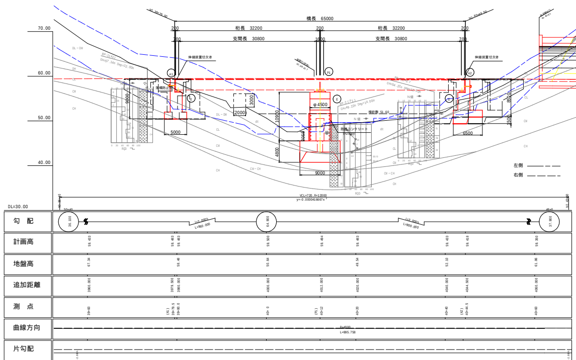
側面図 S=1:300
