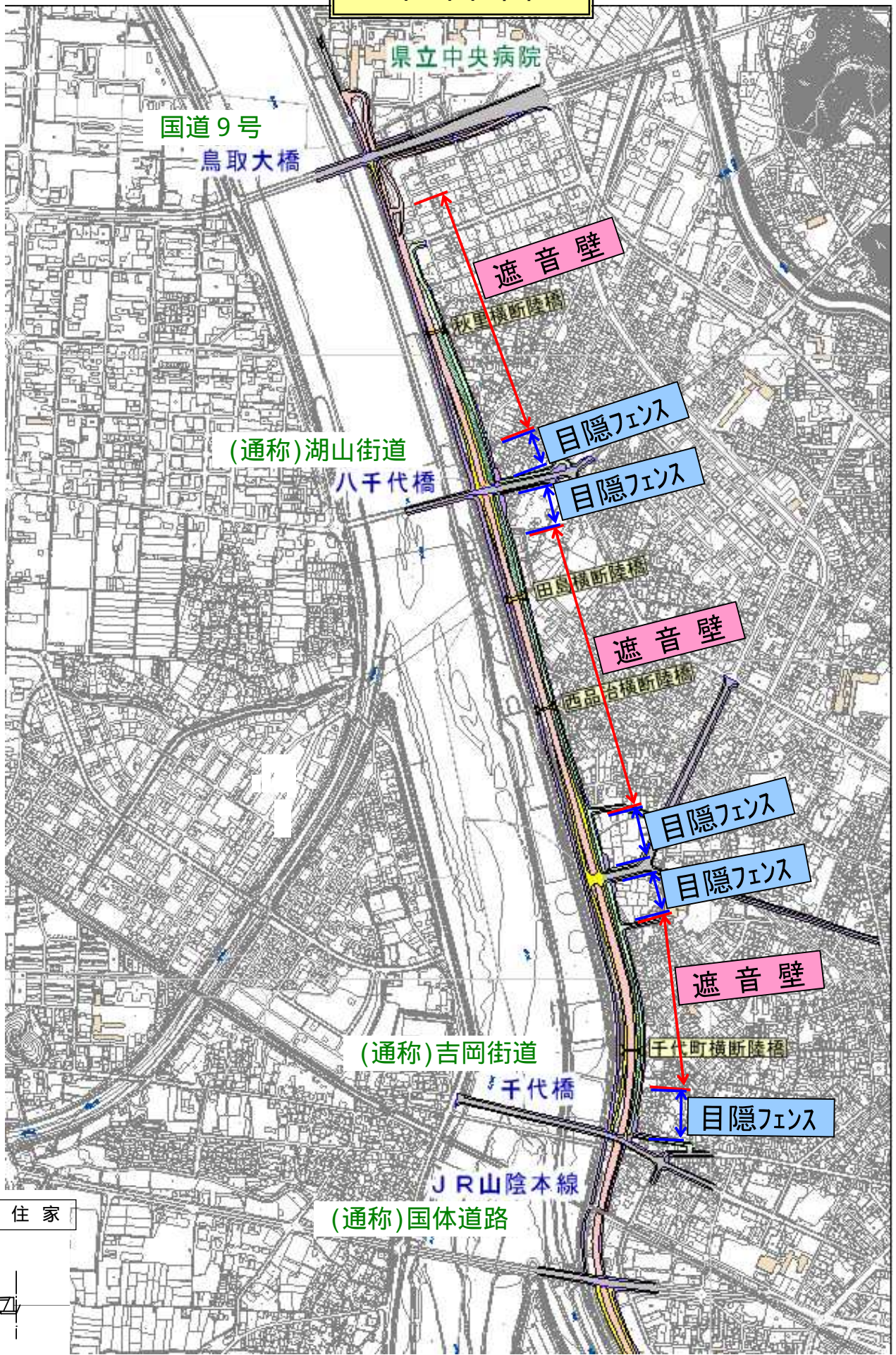
平面図
