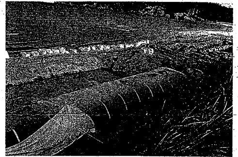
浦富海岸で行われている「サンドバック工法」による浜崖後退の防止事業。1バックが砂160トン。
