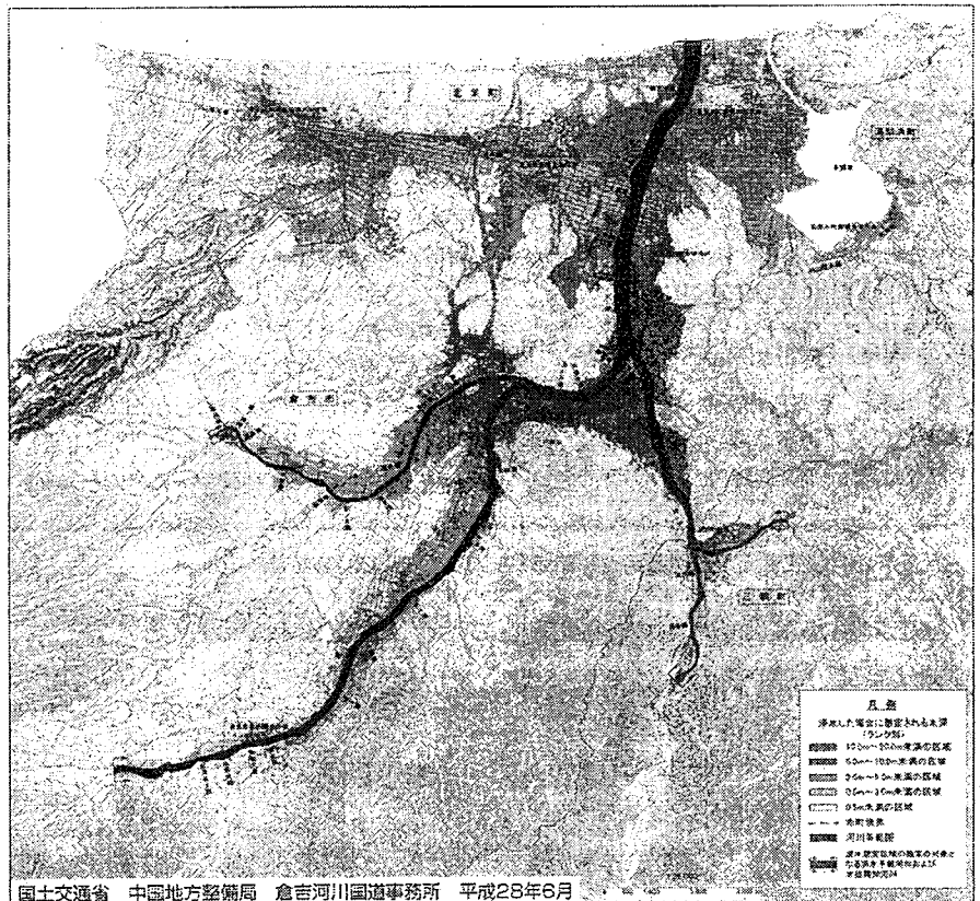
天神川水系洪水浸水想定区域図(想定最大規模)
