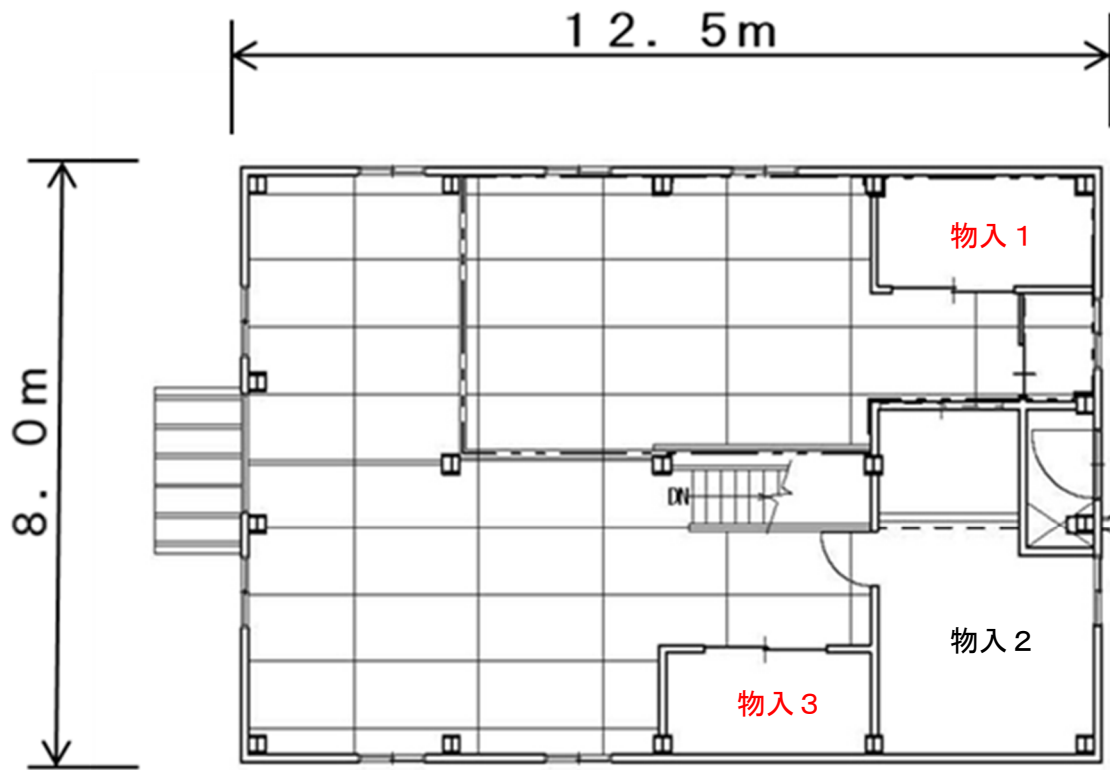
2階図面
