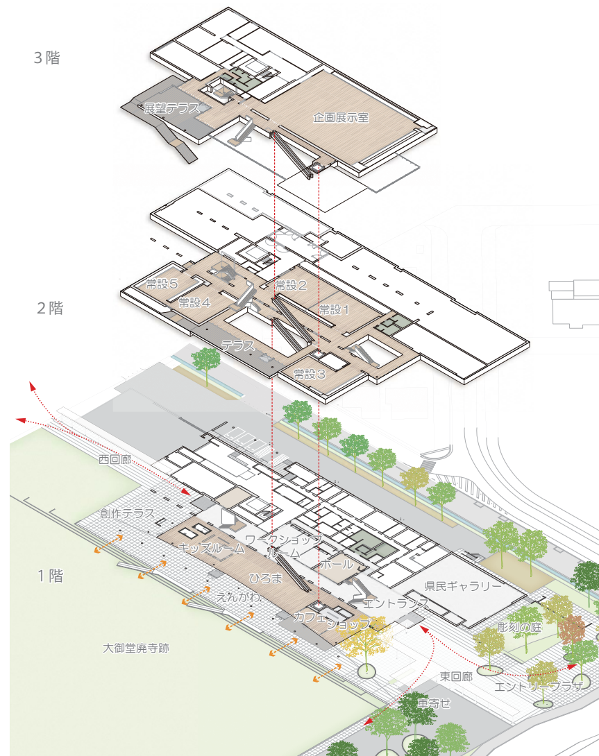
建物構成
