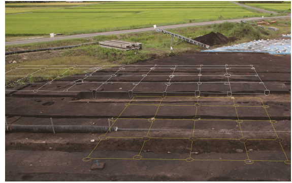
大型建物跡検出状況（北から）
