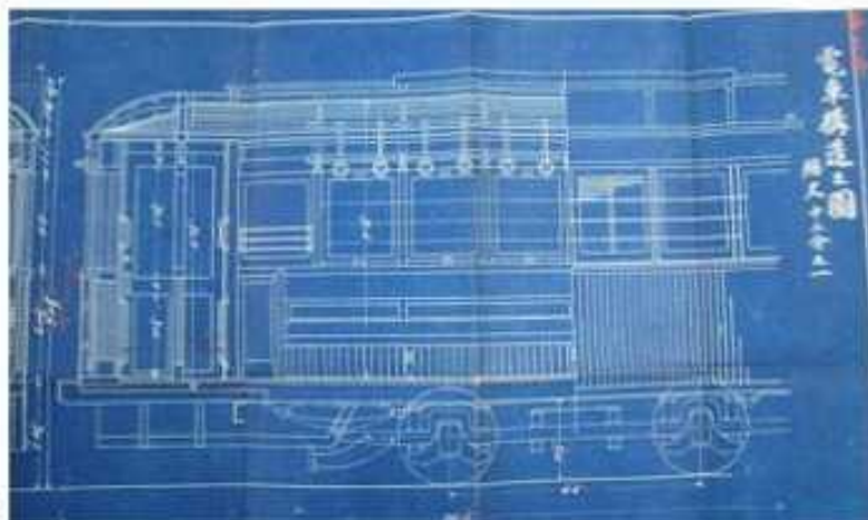
米子電車軌道の車輛図面〈大正15年〉 （国立公文書館蔵）
