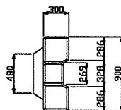
側面図
