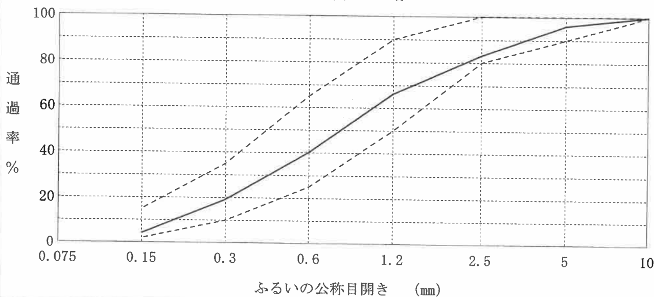
粒 度 曲 線
