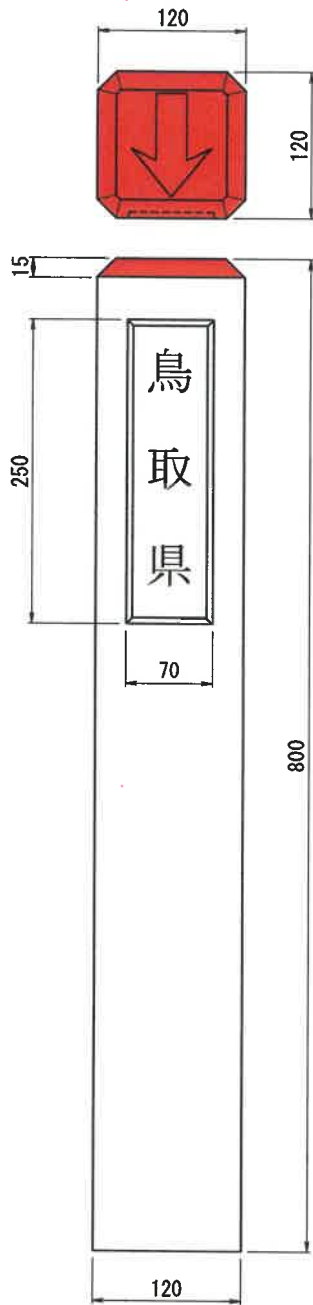
寸法図（中央）
