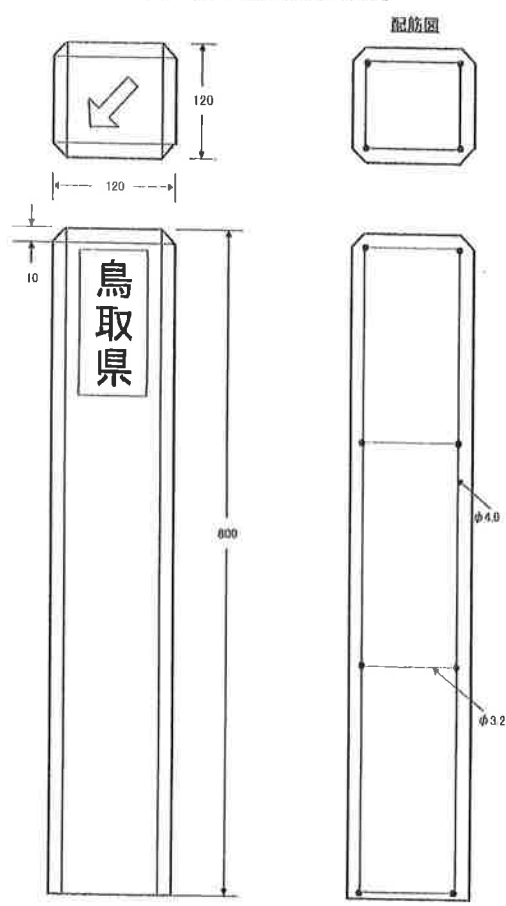
コンクリート境界標柱 (左)
