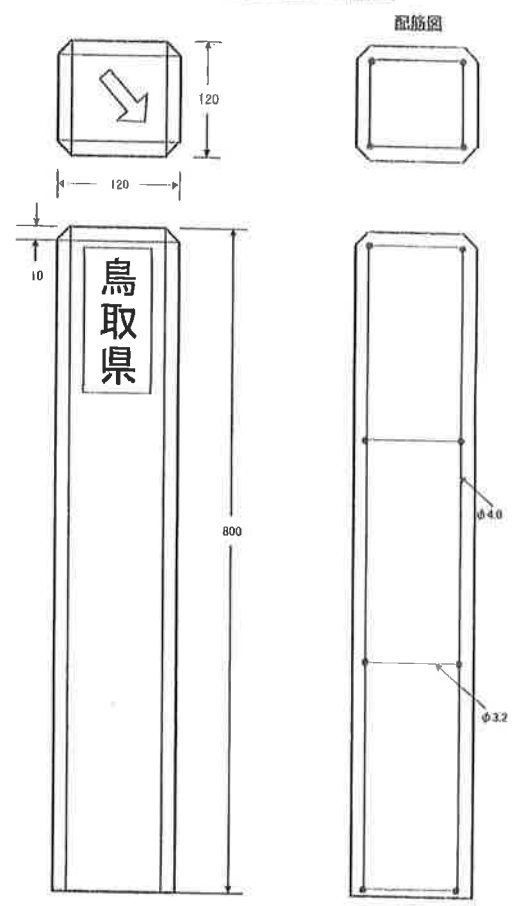
コンクリート境界標柱 (右)
