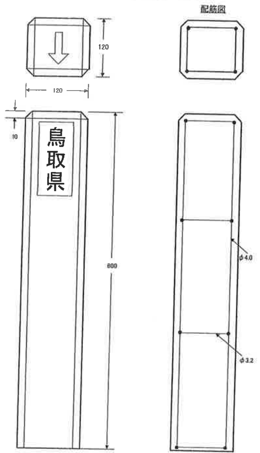
コンクリート境界標柱 (中央)
