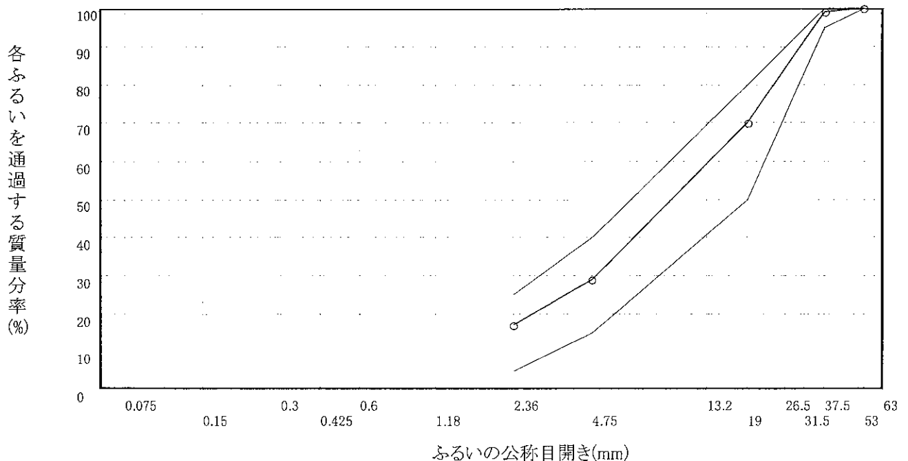
粒度曲線
