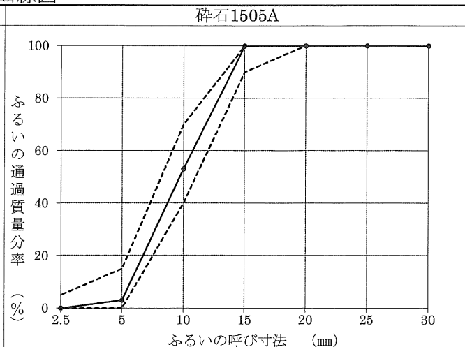
粒度曲線図
