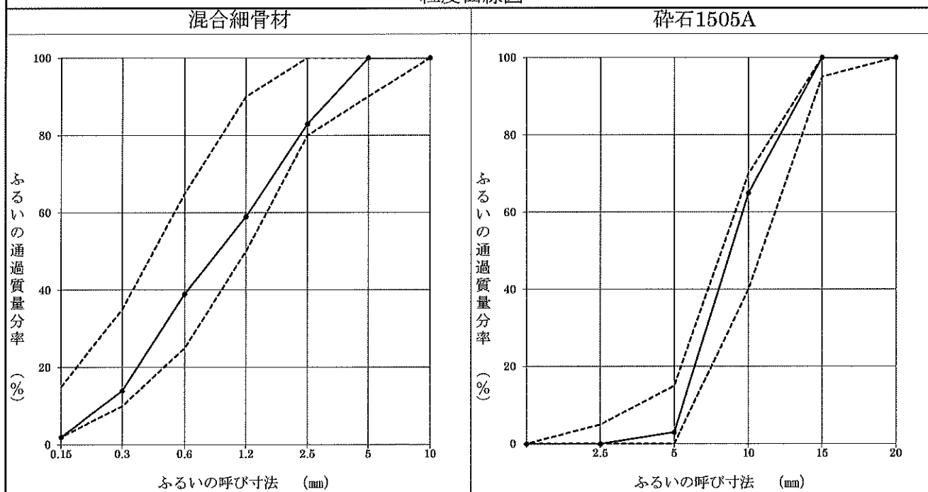
粒度曲線図
