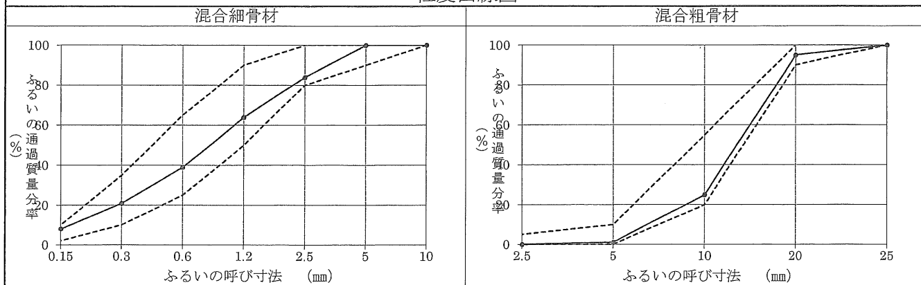
粒度曲線図
