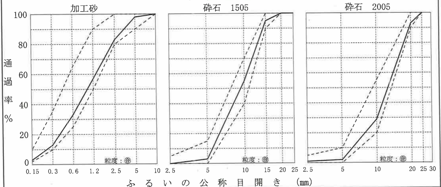
粒 度 曲 線
