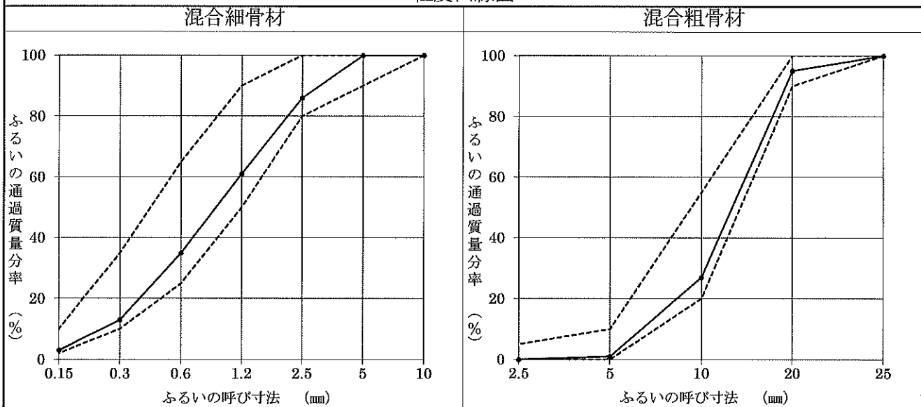
粒度曲線図
