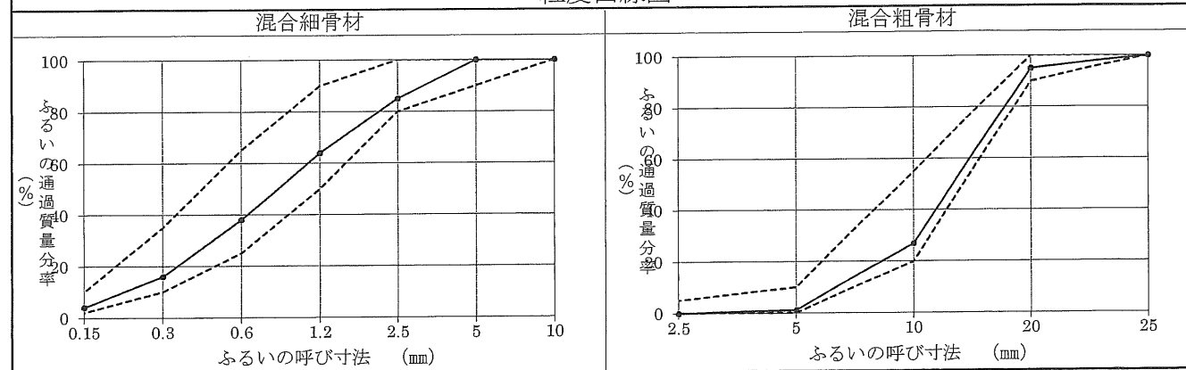
粒度曲線図
