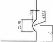
A部詳細図
