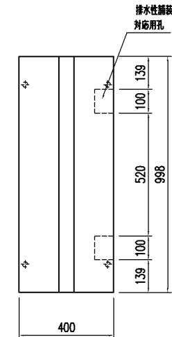
排水性舗装対応孔位置 (FI, S1CI, S2I, RI, NI, OI, BFII)
