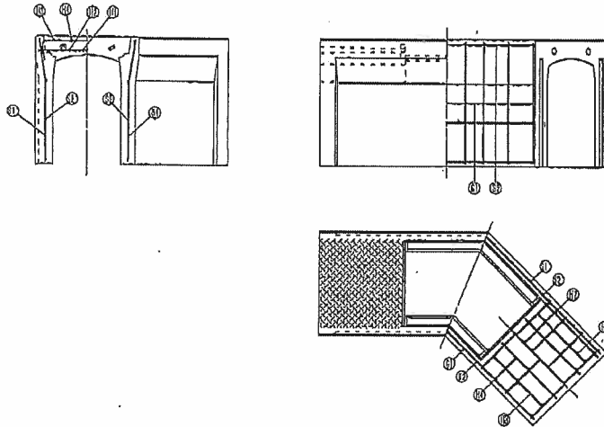
CH-II 可変側溝 コーナー用 135°
