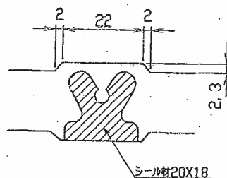
目地部詳細図 (S=1/1)
