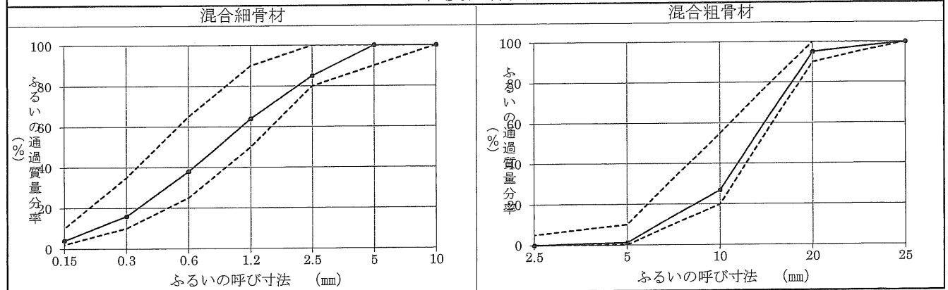
粒度曲線図
