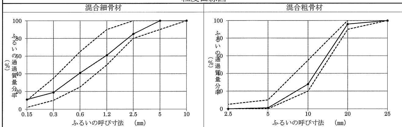
粒度曲線図
