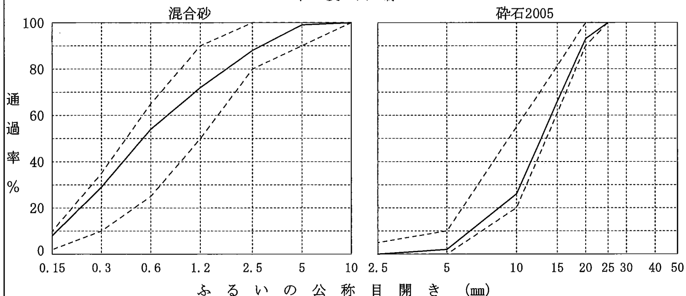
粒 度 曲 線
