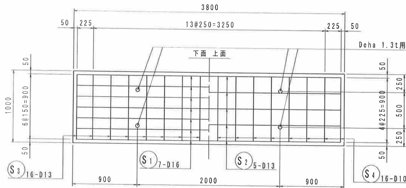
平面図
