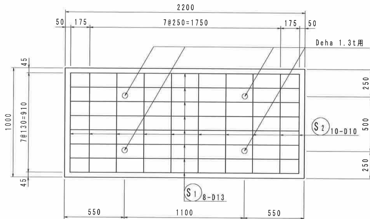
平面図
