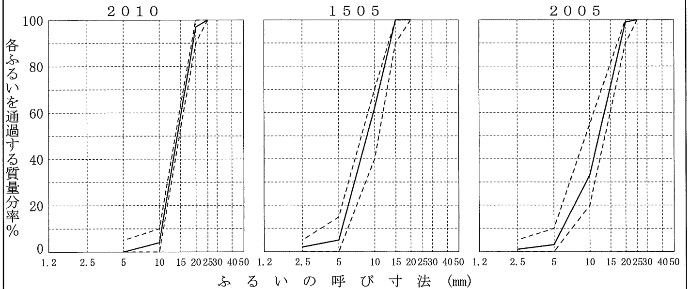
粒 度 曲 線
