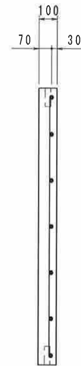
側面図
