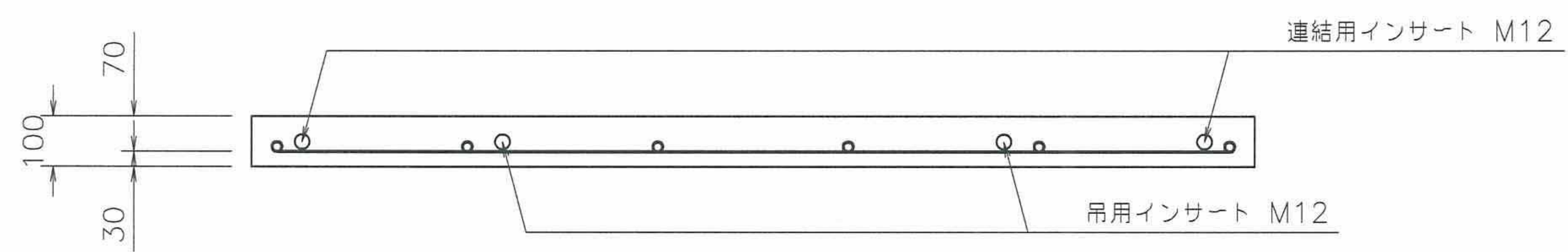
断面図
