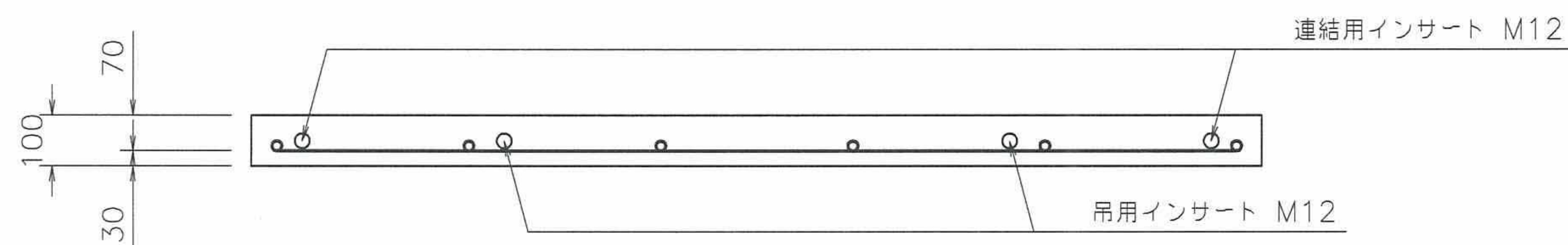
断面図
