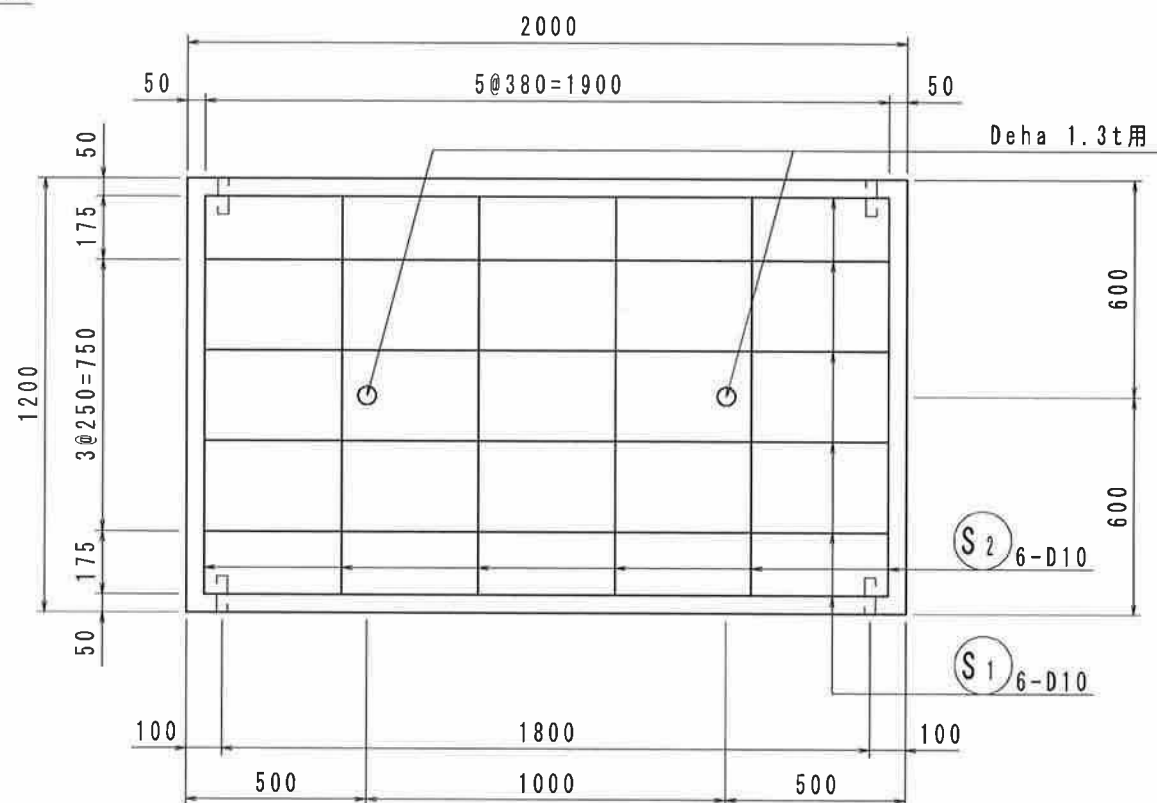
平面図
