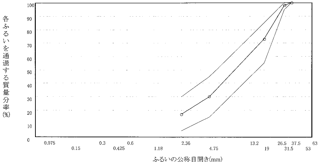
粒度曲線
