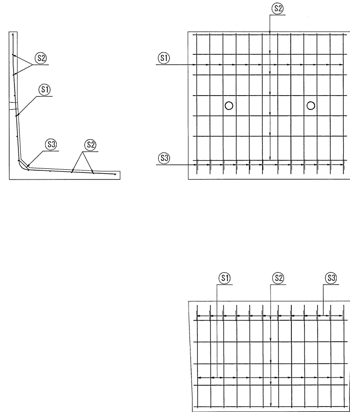
配筋図
