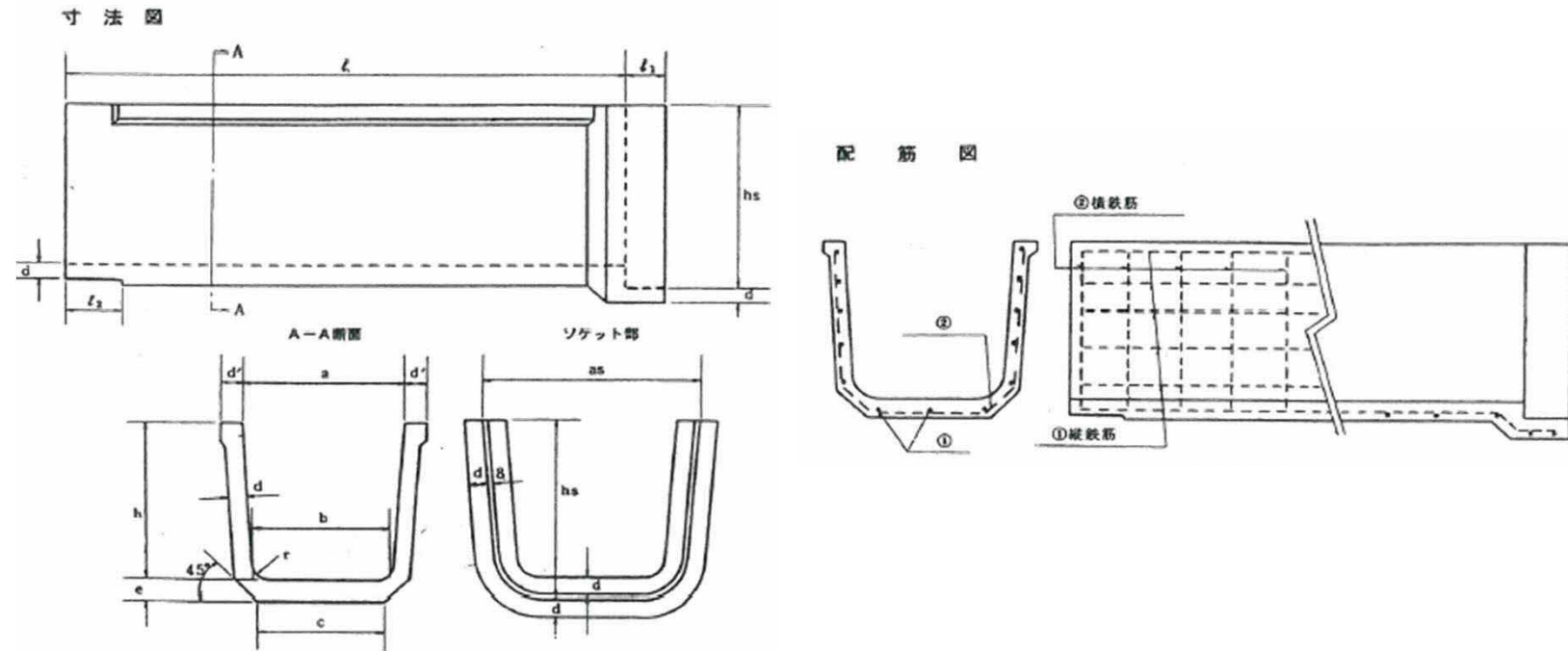
寸法表
