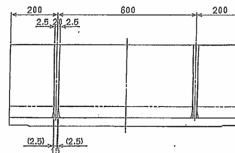
断面図B-B
