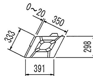
側面図
