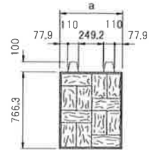
◇正面図
