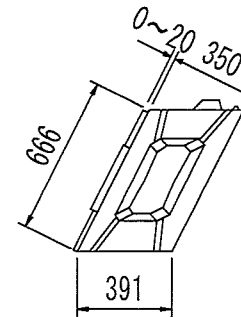
側面図
