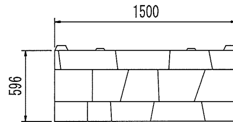
正面図
