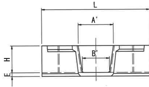
A-A 断面
