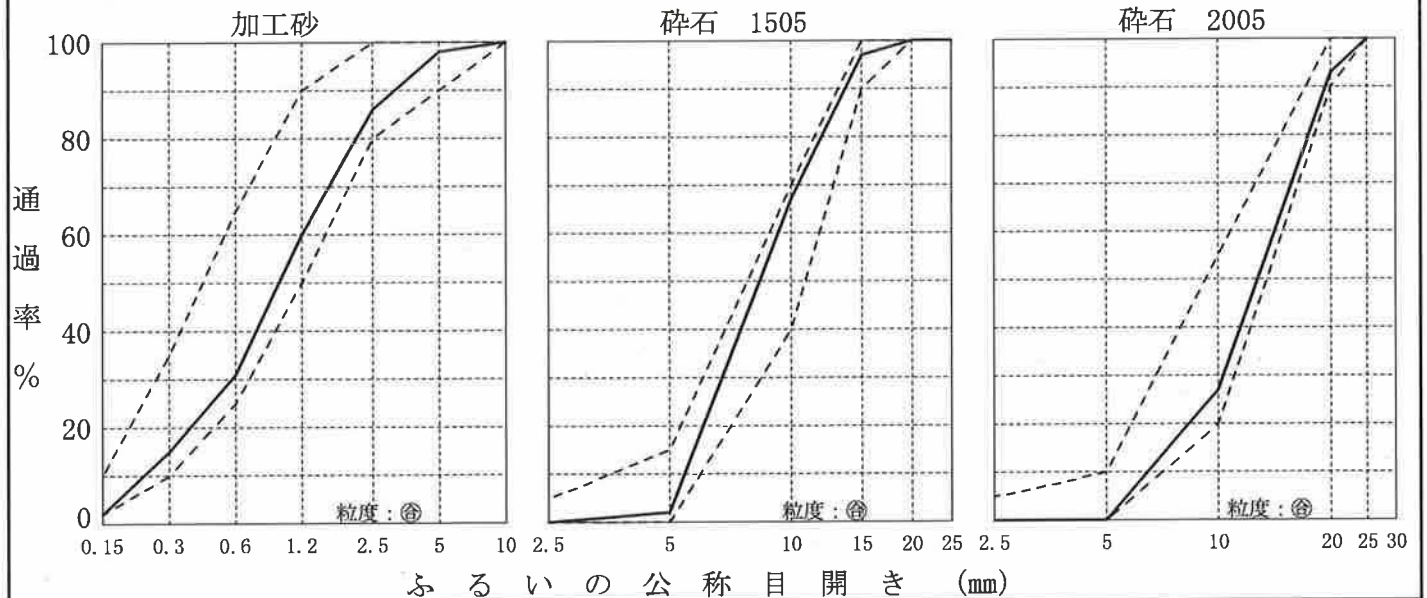
粒 度 曲 線
