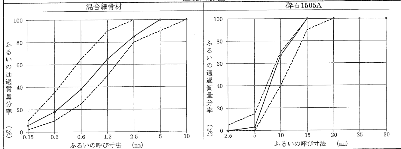
粒度曲線図
