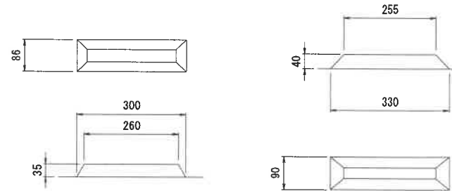
凸部詳細
