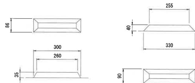
凸部詳細
