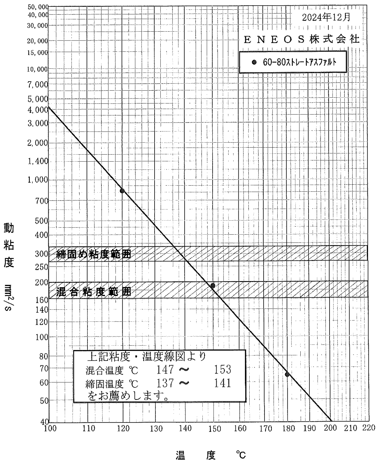
粘度 - 温度図
