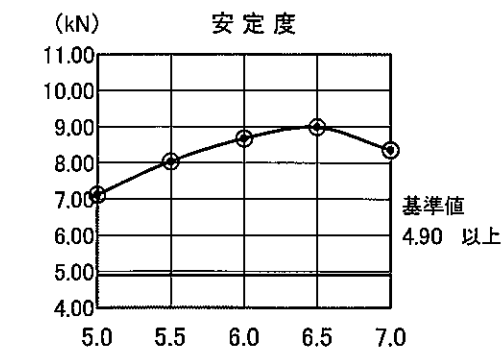
設計アスファルト量の設定図
